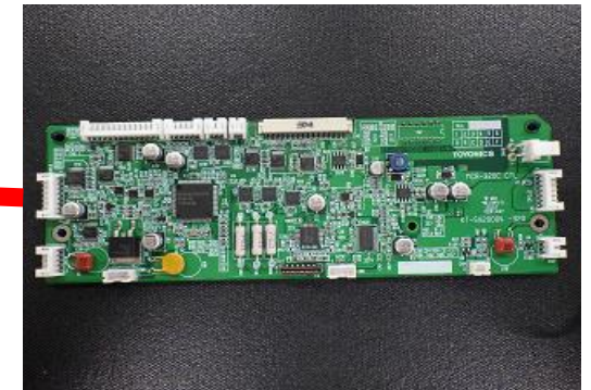
日圧製コネクタ使用TCT-217X CNT基板
