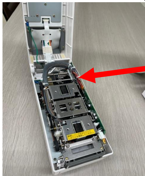
JAE製コネクタ使用TCT-217X CNT基板
